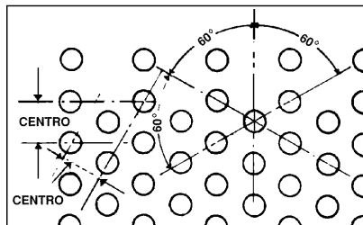
Formación escalonada con ángulo de 60° entre perforación.
